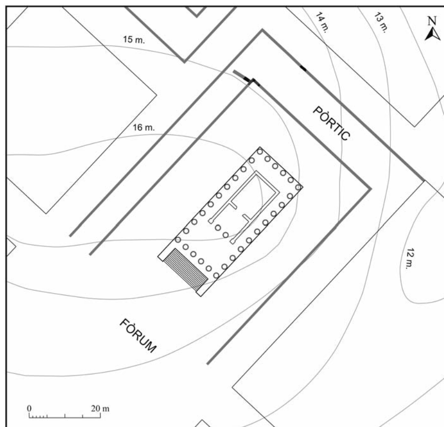
Figura 4 Planta de la terrassa superior del fòrum amb estructures arqueològiques conservades del pòrtic. [Dibuix: MUHBA]
