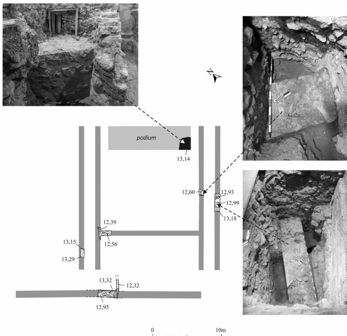
Figura 16 Planta de les estructures conservades sota la basílica dels Sants Màrtirs Just i Pastor i el seu entorn immediat [Hipòtesi: J. Beltrán de Heredia. Planimetria: I. Camps]
